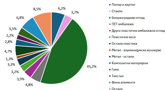
САСТАВ КОМУНАЛНОГ ОТПАДА, 2023. ГОДИНА
